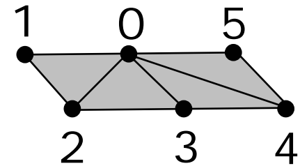
GL_TRIANGLE_FAN
