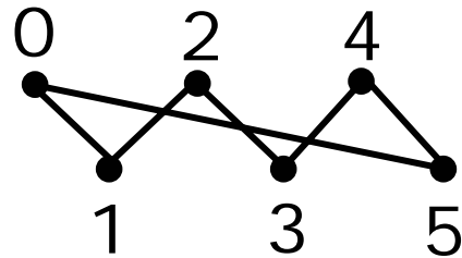
GL_LINE_LOOP
