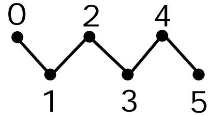
GL_LINE_STRIP
