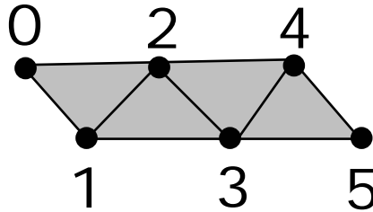
GL_TRIANGLE_STRIP
