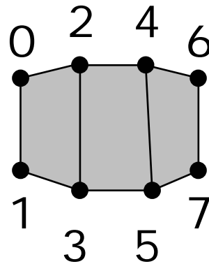
GL_QUAD_STRIP
