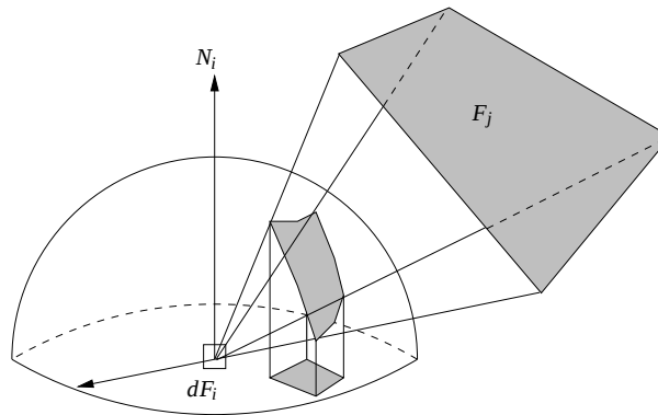
Abbildung 23.2: Geometrische Interpretation des Formfaktors
