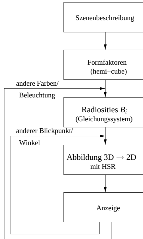
Abbildung 23.4: Ablaufschema beim Radiosityverfahren
