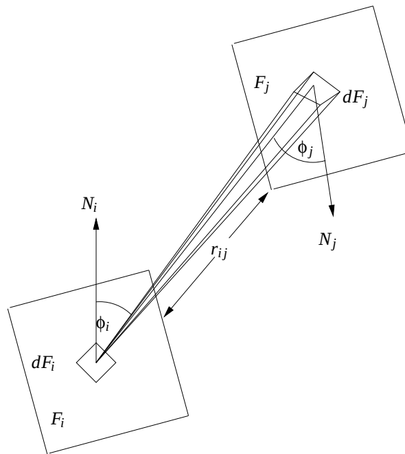
Abbildung 23.1: Der Berechnung von Formfaktoren zugrundeliegende Geometrie
